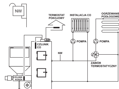
Rys.5. Sterowanie kotłem podajnikowym z jednym obiegiem grzewczym sterowanym termostatem pokojowym, ogrzewaniem podłogowym sterowanym zaworem termostacyjnym.
