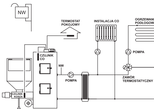
Rys.6. Sterowanie kotłem podajnikowym z jednym obiegiem grzewczym sterowanym termostatem pokojowym, ogrzewaniem podłogowym sterowanym zaworem termostacyjnym. Wymiennik płytowy do rozdziału układu otwartego i zamkniętego.
